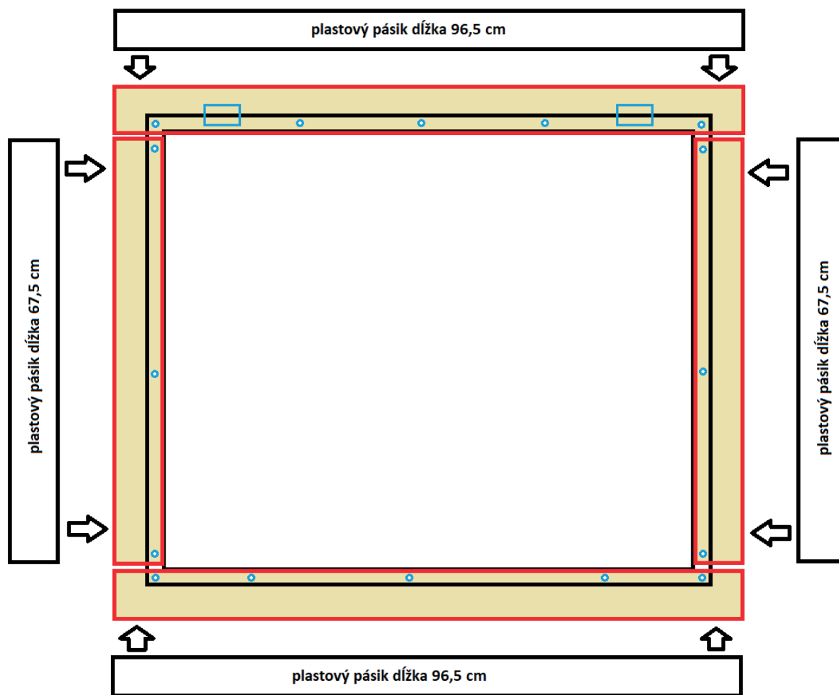
Obrázok 3 – umiestenie skrutiek
